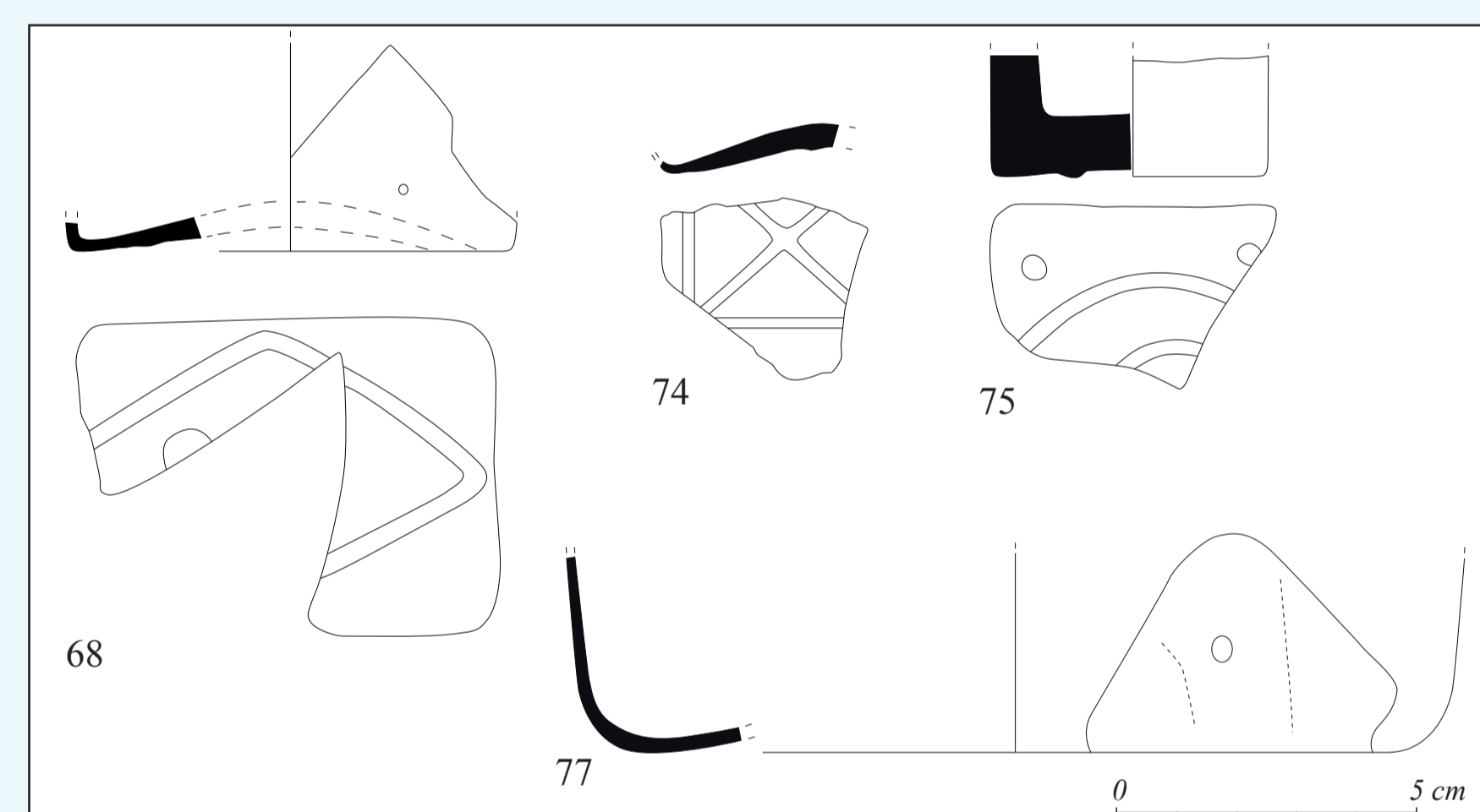
Récipients de stockage (DAO A. Lacroix, éch. 1/2)
