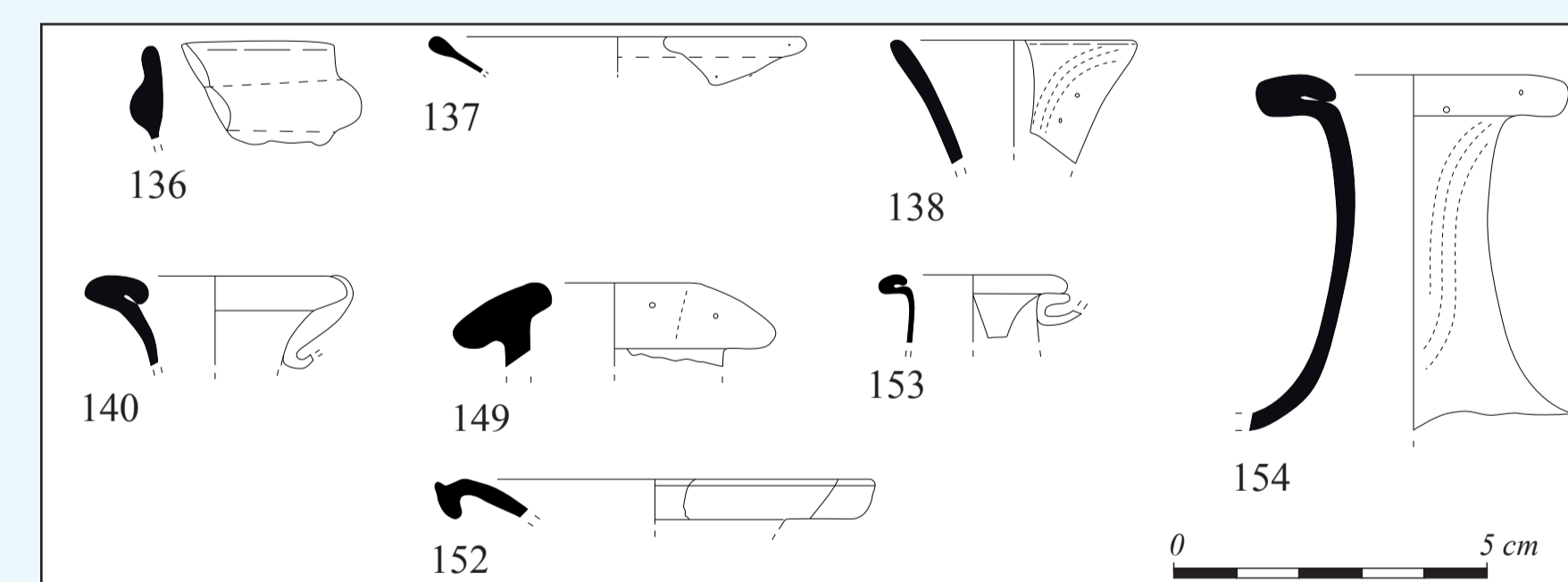
Bords de récipient (DAO A. Lacroix, éch. 1/2)
